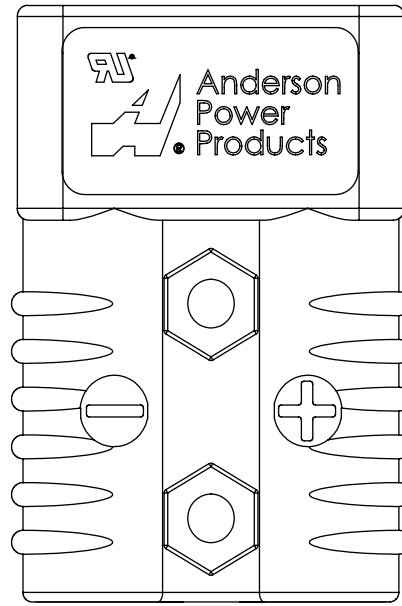
SB® 175 - 2 Pole
